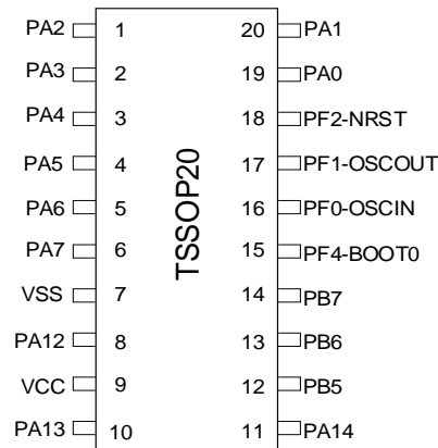
图 4-8 TSSOP20 Pinout2 DM32F030F2xP表 4-1
